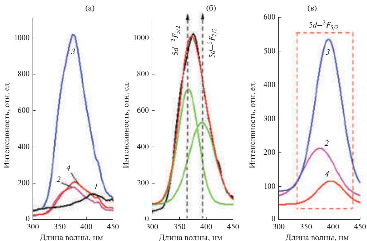
Рис. 7. Спектры ФЛ порошков Се-ТКФ после синтеза: а – общий вид спектров, б – спектр ТКФ-2 после аппроксимации на два пика, в – спектры перехода 5d \rightarrow 2F_{5/2} ; 1 – ТКФ-0, 2 – ТКФ-1, 3 – ТКФ-2, 4 – ТКФ-3.
