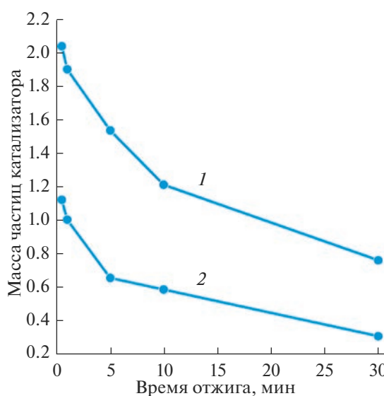
Рис. 4. Изменение суммарной массы наночастиц катализатора за время отжига при 700 (1), 800°C (2).
